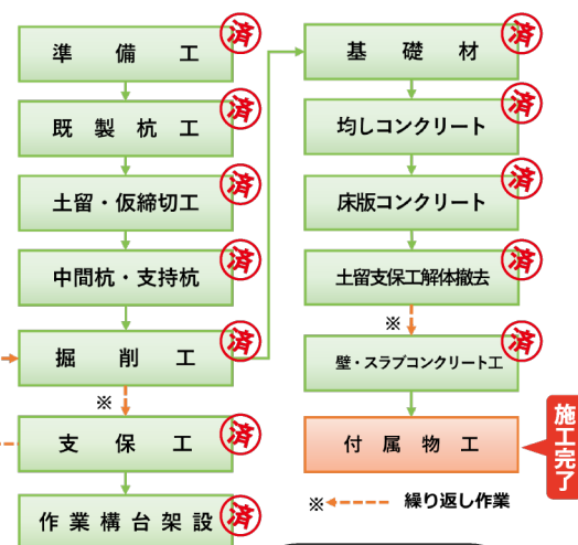
フロー図
