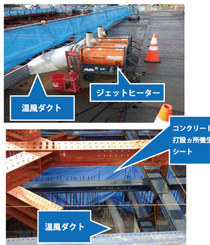
底版コンクリート養生状況
