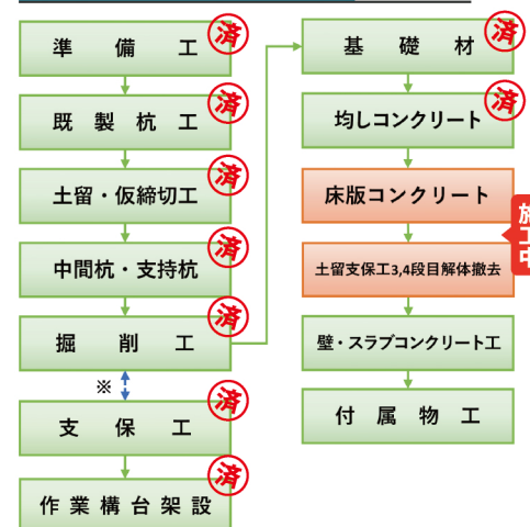
フロー図
