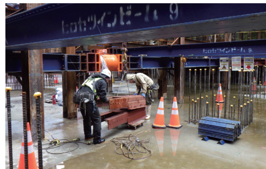
土留支保工一部解体
