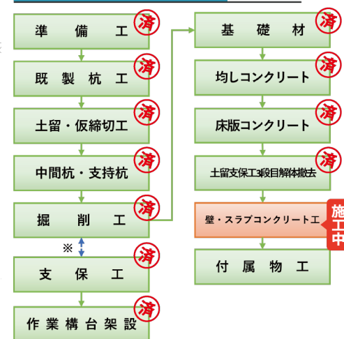
フロー図
