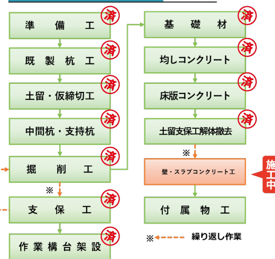
フロー図
